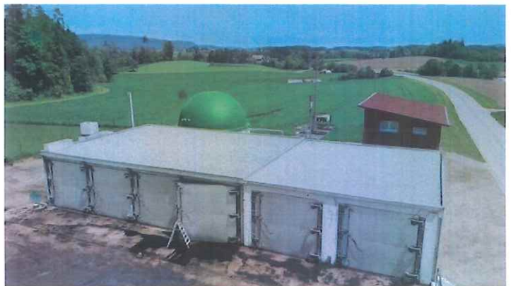
Schaubild 1: Bild einer solchen Feststoffbiogasanlage (© renergon-biogas.com)
